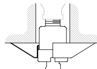
Type E Escutcheon/ Подрозетник/ Rozet
